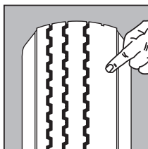
Usure irrégulière des épaulements (faire inspecter)
