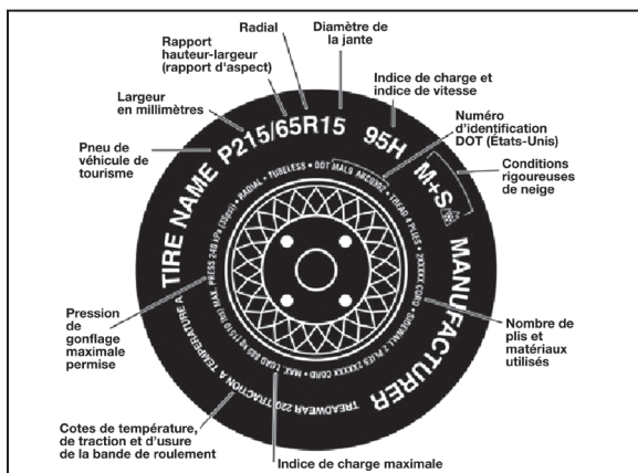
Illustration 3 : Inscriptions types d'un pneu tourisme
