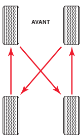
Véhicules à quatre roues motrices et à traction arrière
