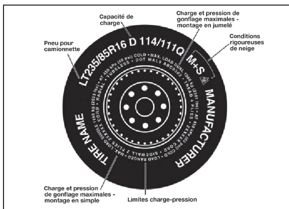
Illustration 4 : Inscriptions types d'un pneu pour camionnette
