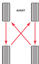
Véhicules à traction avant
